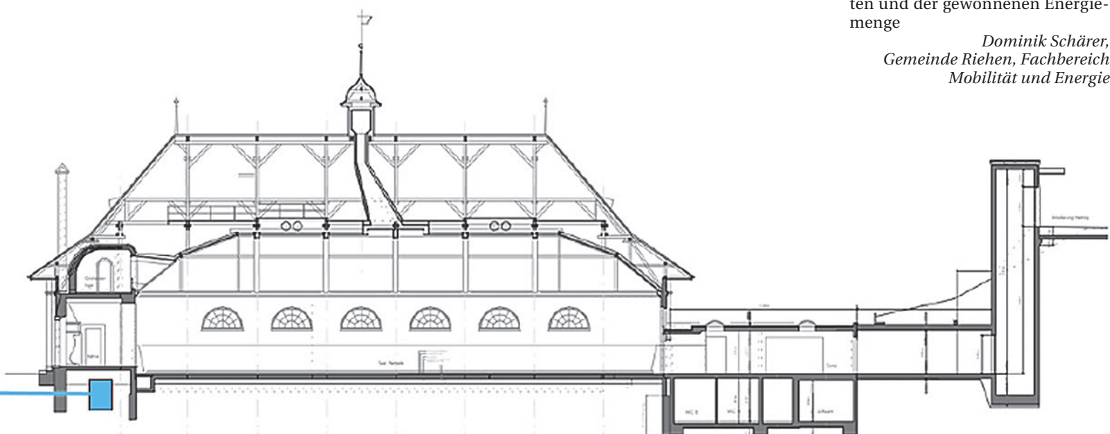
Das Prinzip Erdkörbe mit Wärmepumpe am Beispiel der Reithalle Wenkenhof.
