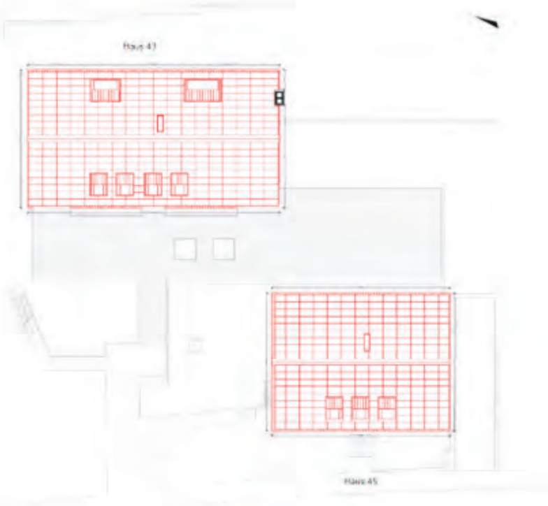
Der Dachaufsichtsplan der Fotovoltaikanlage Rainallee 43/45, die im Rahmen der laufenden Sanierung installiert wird.
